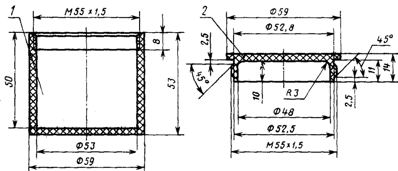
1 — чашка фторопластовая; 2 — навинчивающаяся крышка
